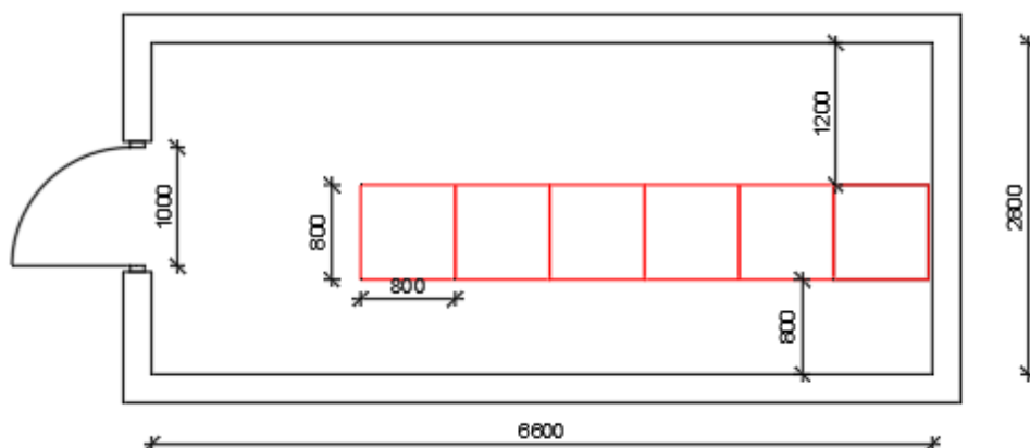
Fig.02: Typisk layout kommunikasjonsrom
